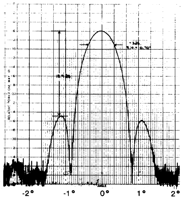
H-Plane — W-Band (12" Dia.)
