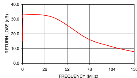
ADT8-1T INPUT RETURN LOSS
