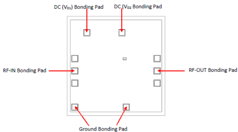
Fig 2. Die Layout
