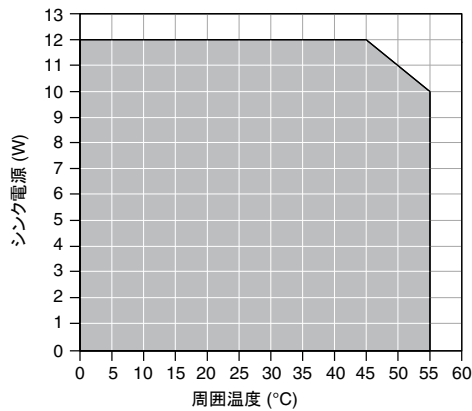
図 4. 周囲温度によるシンク電源の低下
