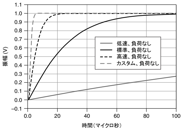
図 5. 1 mA レンジ、負荷なしステップ応答 (標準)
