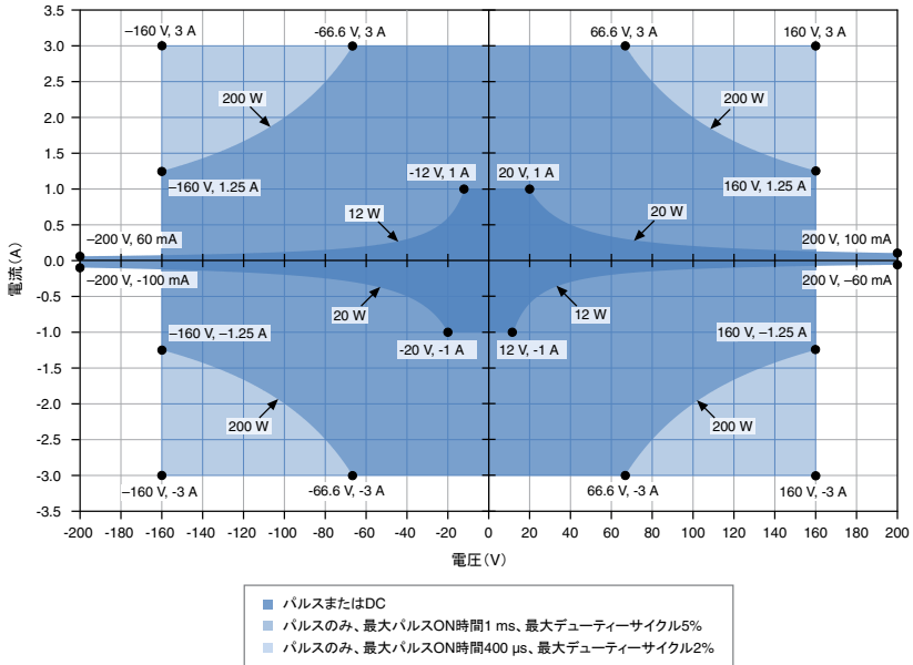
図 1. 象限図 4
