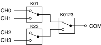
図 4. NI 2594 電源投入時の状態
