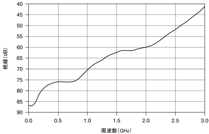
図 3. 標準絶縁
