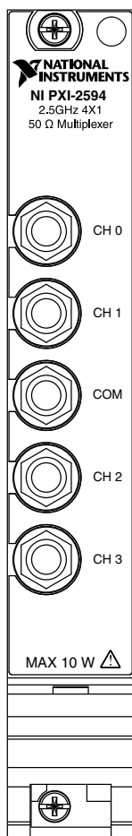
図 5. NI 2594 フロントパネルのネクタピン配列
