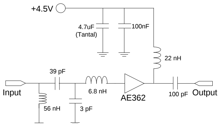
EVB BOM
