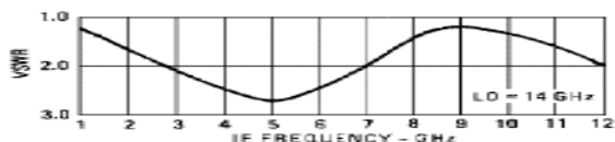
I-Port VSWR
