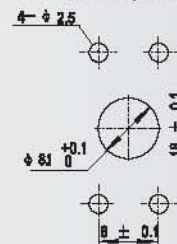
安装开孔尺寸 Mounting hole
