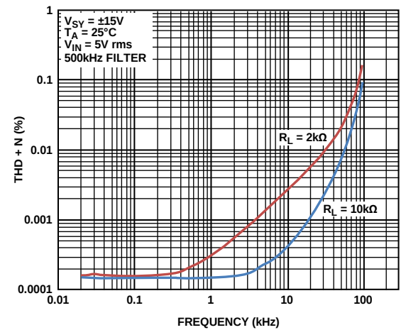
图98. THD + N与频率的关系，500 kHz滤波器
