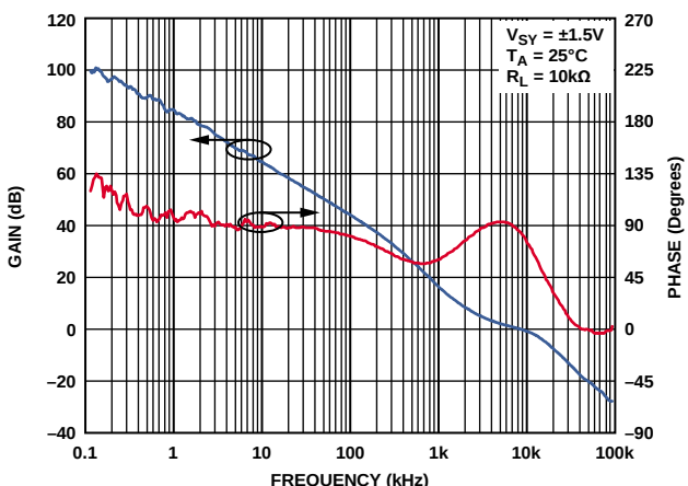
图23. 开环增益和相位与频率的关系
