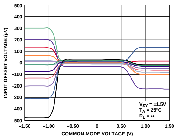
图17. 输入失调电压与共模电压的关系
