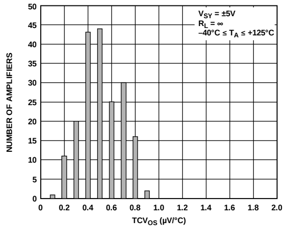
图45. TCV_{OS} 分布图(SOIC、MSOP和TSOP)
