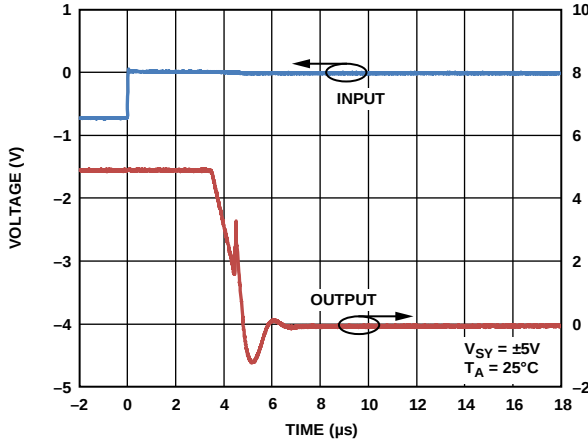
图70. 正50%过载恢复时间
