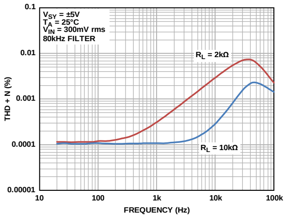
图68. THD + N与频率的关系，80 kHz滤波器
