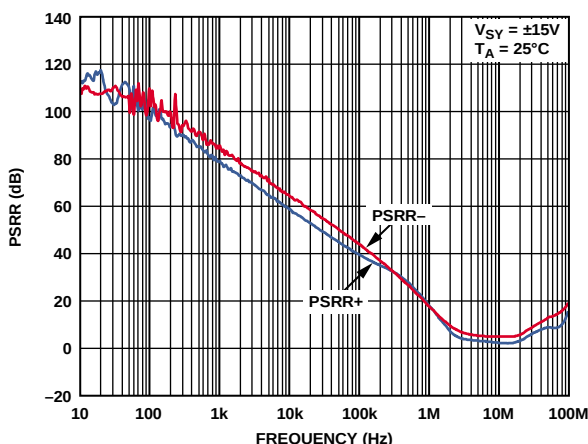
图88. PSRR与频率的关系
