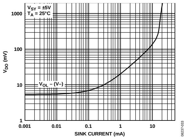
图53. 压差( V_{DO} )与吸电流的关系
