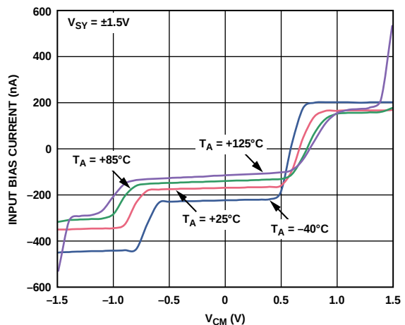
图20. 不同温度下输入偏置电流与 V_{CM} 的关系
