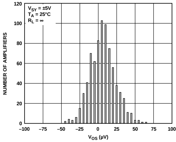
图41. 输入失调电压( V_{OS} )分布图(SOIC)
