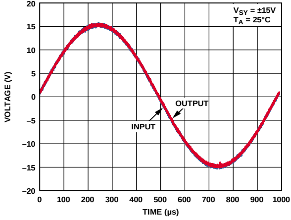
图100. 无相位反转
