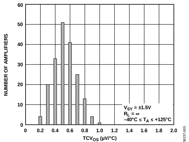
图14. TCV_{OS} 分布图(SOIC、MSOP和TSSOP)
