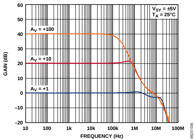
图55. 闭环增益与频率的关系
