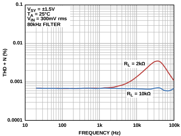
图37. THD + N与频率的关系，80 kHz滤波器
