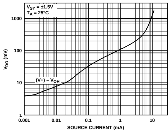
图21. 压差( V_{D0} )与源电流的关系
