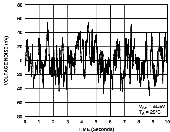
图33. 电压噪声(0.1 Hz至10 Hz)
