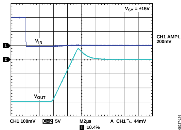
图102. 负50%过载恢复时间
