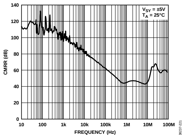
图58. CMRR与频率的关系
