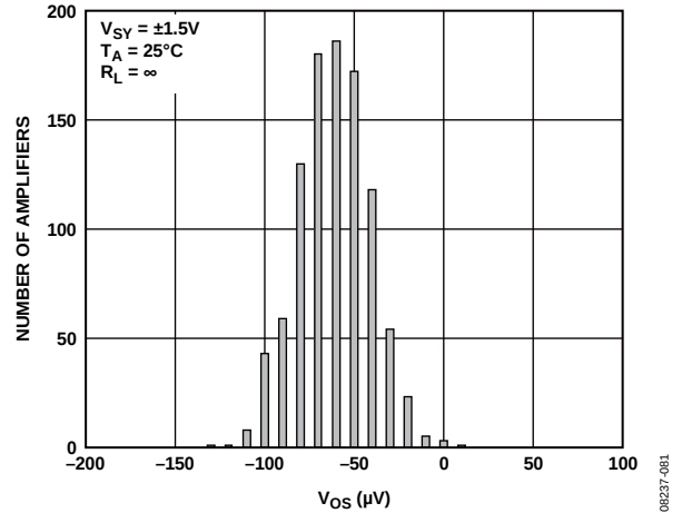
图13. 输入失调电压( V_{OS} )分布图(LFCSP)
