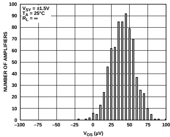
图11. 输入失调电压( V_{OS} )分布图(SOT-23)
