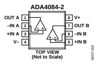
图7. ADA4084-2, 8引脚 SOIC (R)
