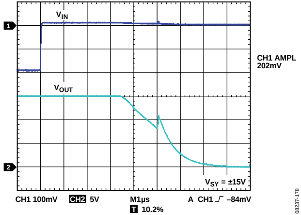
图101. 正50%过载恢复时间
