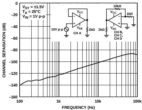
图34. 通道隔离与频率的关系
