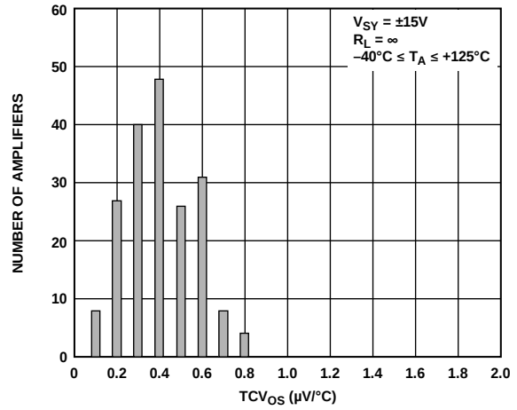
图76. TCV_{OS} 分布图(SOIC、MSOP和TSOP)
