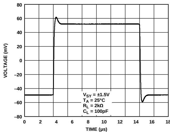
图29. 小信号瞬态响应
