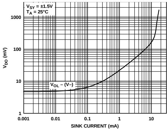
图22. 压差( V_{DO} )与吸电流的关系
