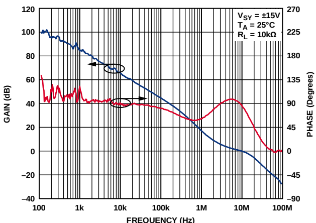
图85. 开环增益和相位与频率的关系
