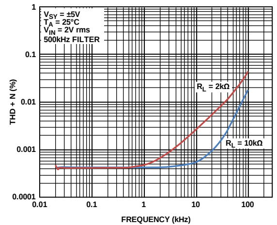
图67. THD + N与频率的关系，500 kHz滤波器
