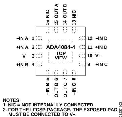
图9. ADA4084-4, 16引脚 LFCSP (CP)
