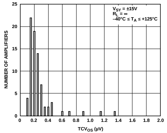
图77. TCV_{OS} 分布图(SOT-23)
