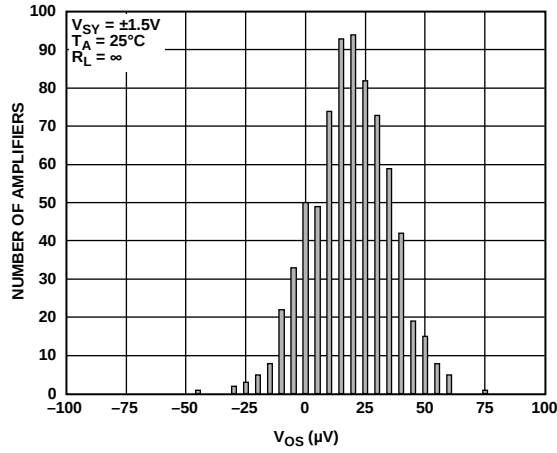
图73. 输入失调电压( V_{OS} )分布图(SOT-23)
