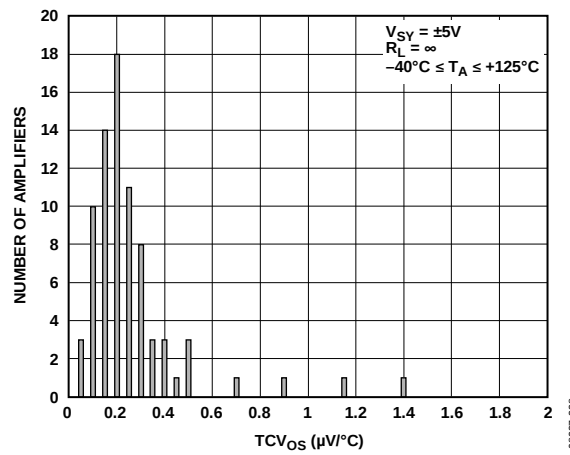
图46. TCV_{OS} 分布图(SOT-23)
