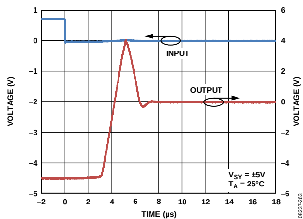
图71. 负50%过载恢复时间
