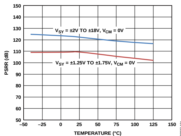
图105. PSRR与温度的关系
