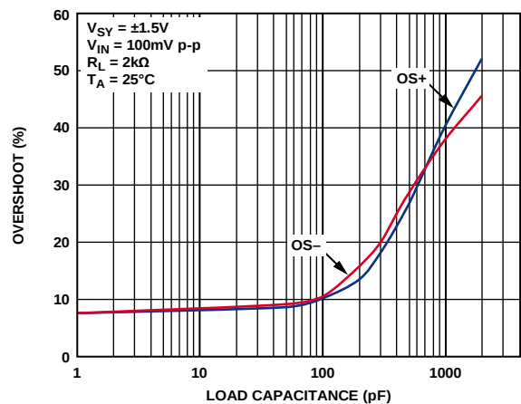
图32. 过冲与负载电容的关系
