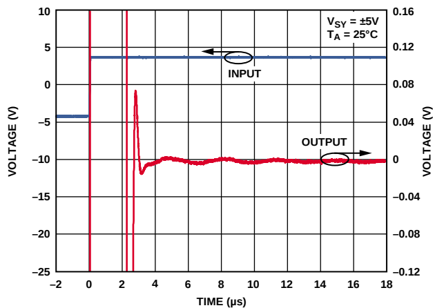
图61. 建立时间
