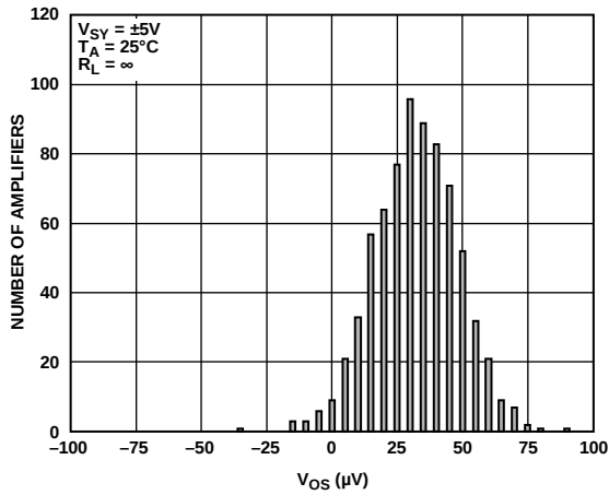
图42. 输入失调电压( V_{OS} )分布图(SOT-23)
