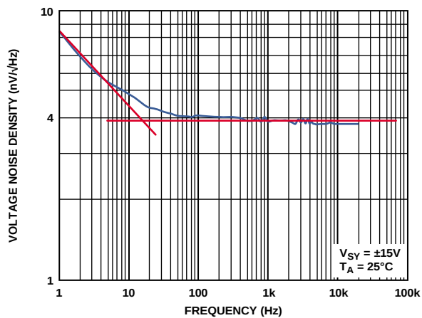
图93. 电压噪声密度与频率的关系
