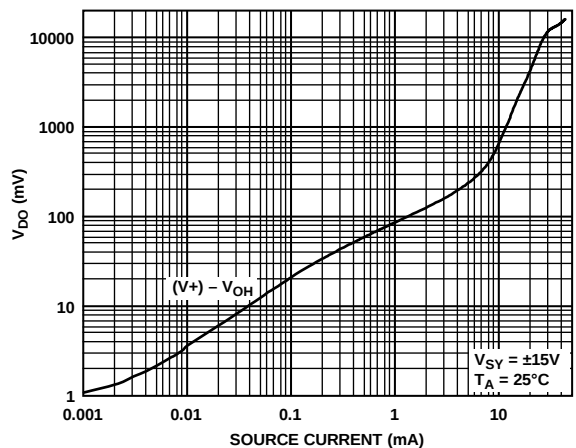
图83. 压差( V_{DO} )与源电流的关系
