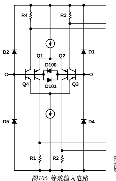
图106. 等效输入电路
