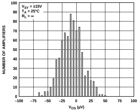
图72. 输入失调电压( V_{OS} )分布图(SOIC)
