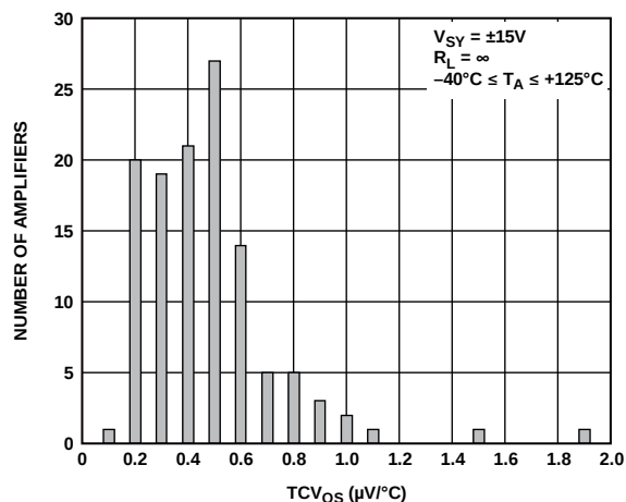
图78. TCV_{0s} 分布图(LFCSP)
