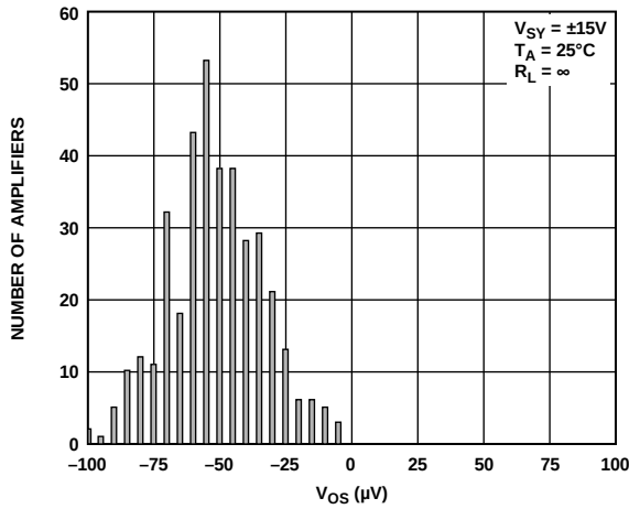
图74. 输入失调电压( V_{OS} )分布图(MSOP和TSOP)
