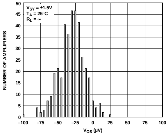
图12. 输入失调电压( V_{OS} )分布图(MSOP和TSSOP)
