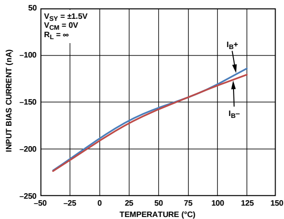
图19. 输入偏置电流与温度的关系
