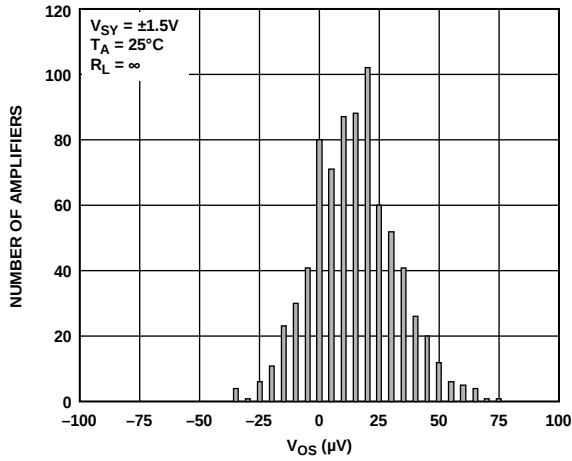
图10. 输入失调电压( V_{OS} )分布图(SOIC)
