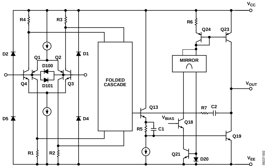
图2. 原理示意图
