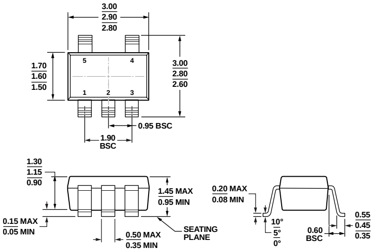
图113. 5引脚小型晶体管封装[SOT-23]
