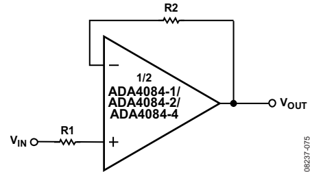
图108. 输入端的串联电阻将过压电流限制在安全值以下
