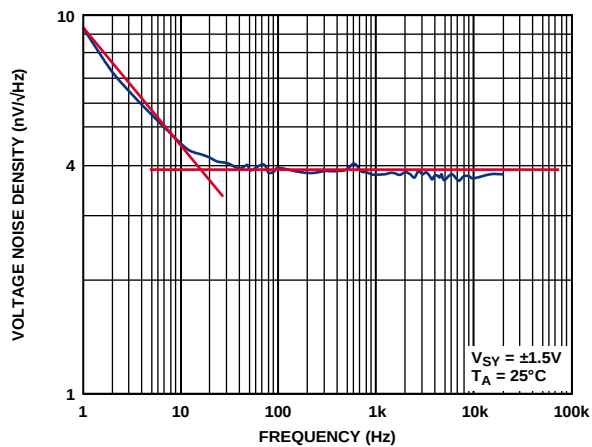
图31. 电压噪声密度与频率的关系
