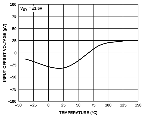
图18. 输入失调电压与温度的关系
