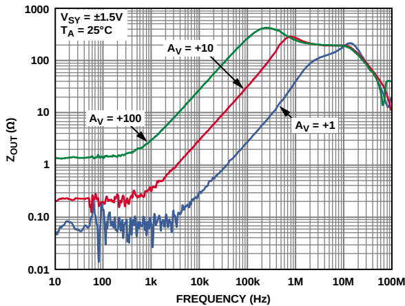
图25. 输出阻抗( Z_{OUT} )与频率的关系
