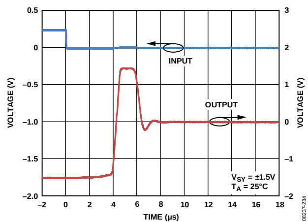
图40. 负50%过载恢复时间
