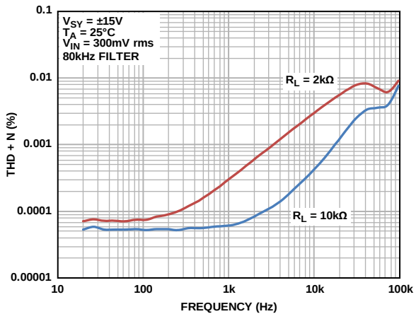
图99. THD + N与频率的关系，80 kHz滤波器
