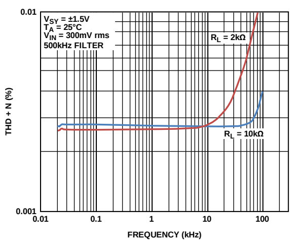
图36. THD + N与频率的关系，500 kHz滤波器
