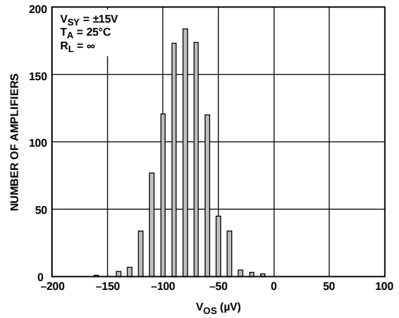
图75. 输入失调电压( V_{OS} )分布图(LFCSP)
