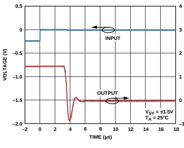
图39. 正50%过载恢复时间
