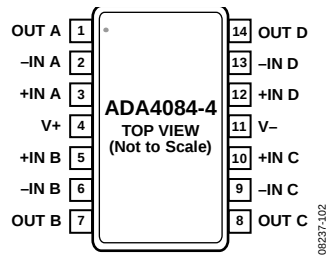
图8. ADA4084-4, 14引脚 TSSOP (RU)
