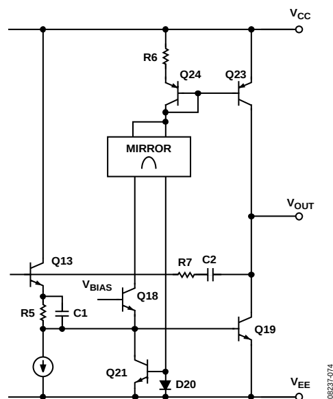
图107. 等效输出电路
