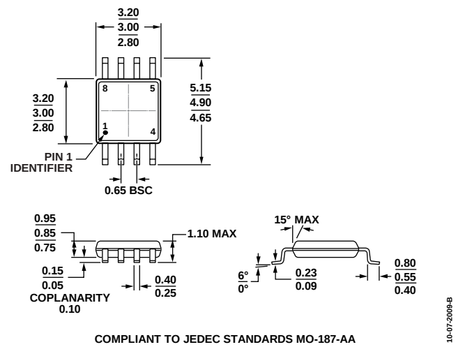
图114. 8引脚超小型封装[MSOP] (RM-8) 图示尺寸单位: mm
