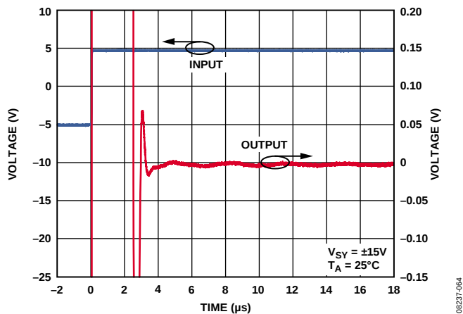
图92. 建立时间
