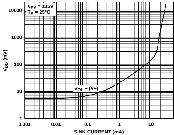
图84. 压差( V_{DO} )与吸电流的关系
