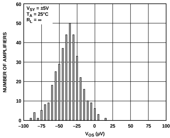
图43. 输入失调电压( V_{OS} )分布图(MSOP和TSOP)
