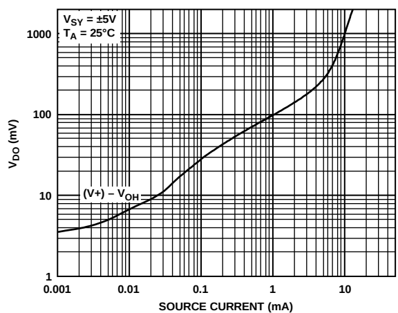
图52. 压差( V_{D0} )与源电流的关系
