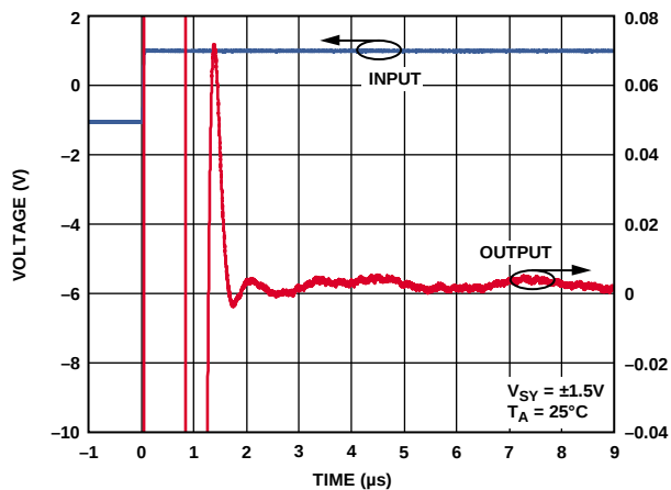
图30. 建立时间
