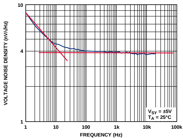
图62. 电压噪声密度与频率的关系
