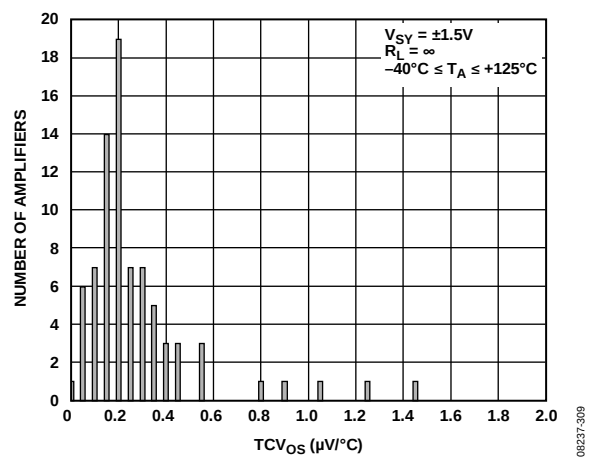
图15. TCV_{OS} 分布图(SOT-23)
