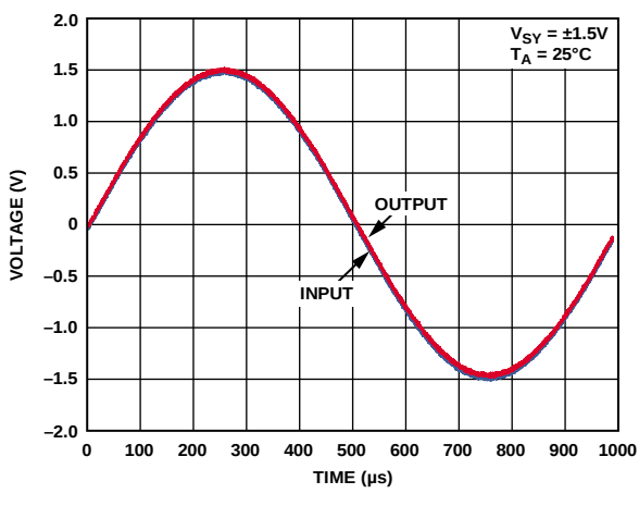
图38. 无相位反转
