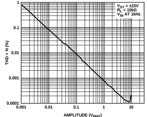
图97. THD + N与幅度的关系
