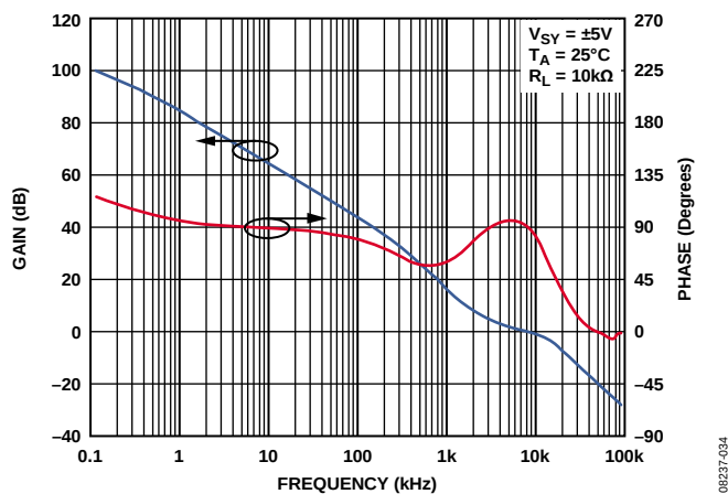
图54. 开环增益和相位与频率的关系
