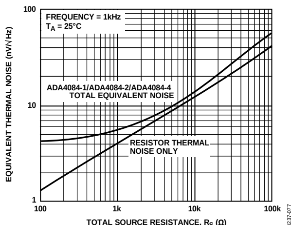
图110. 等效热噪声与总源电阻的关系
