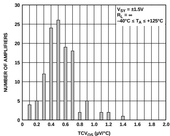
图16. TCV_{0s} 分布图(LFCSP)
