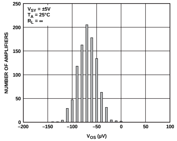
图44. 输入失调电压( V_{OS} )分布图(LFCSP)
