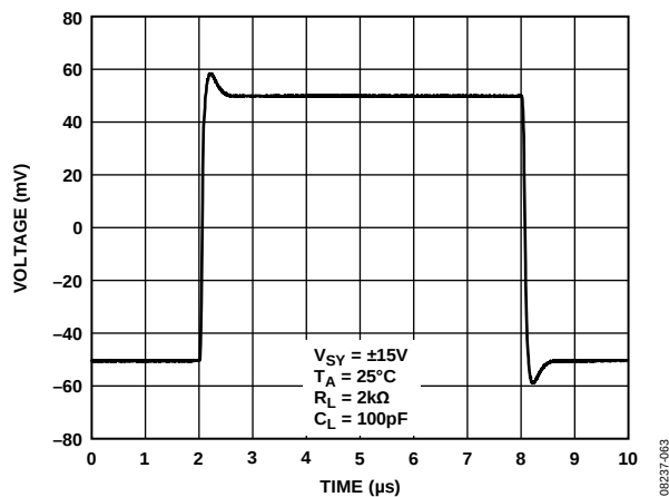
图91. 小信号瞬态响应
