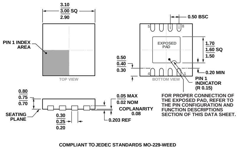
图115. 8引脚引线框芯片级封装[LFCSP_WD] 3 mm × 3 mm, 超薄体, 双排引脚 (CP-8-12) 图示尺寸单位: mm
