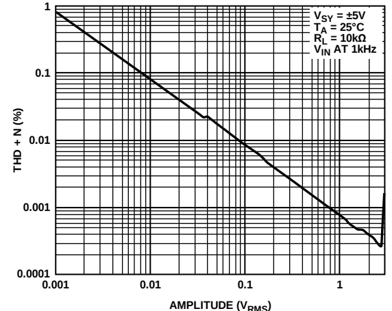
图66. THD + N与幅度的关系
