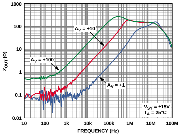
图87. 输出阻抗( Z_{OUT} )与频率的关系
