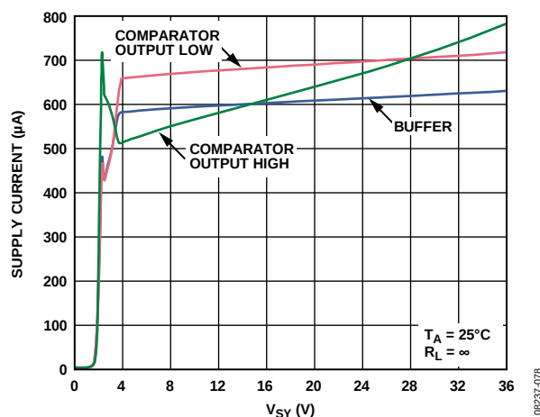
图111. 电源电流与电源电压( V_{SV} )的关系
