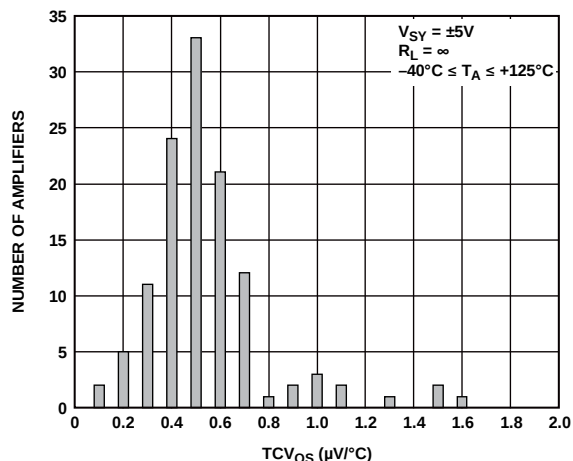
图47. TCV_{0s} 分布图(LFCSP)
