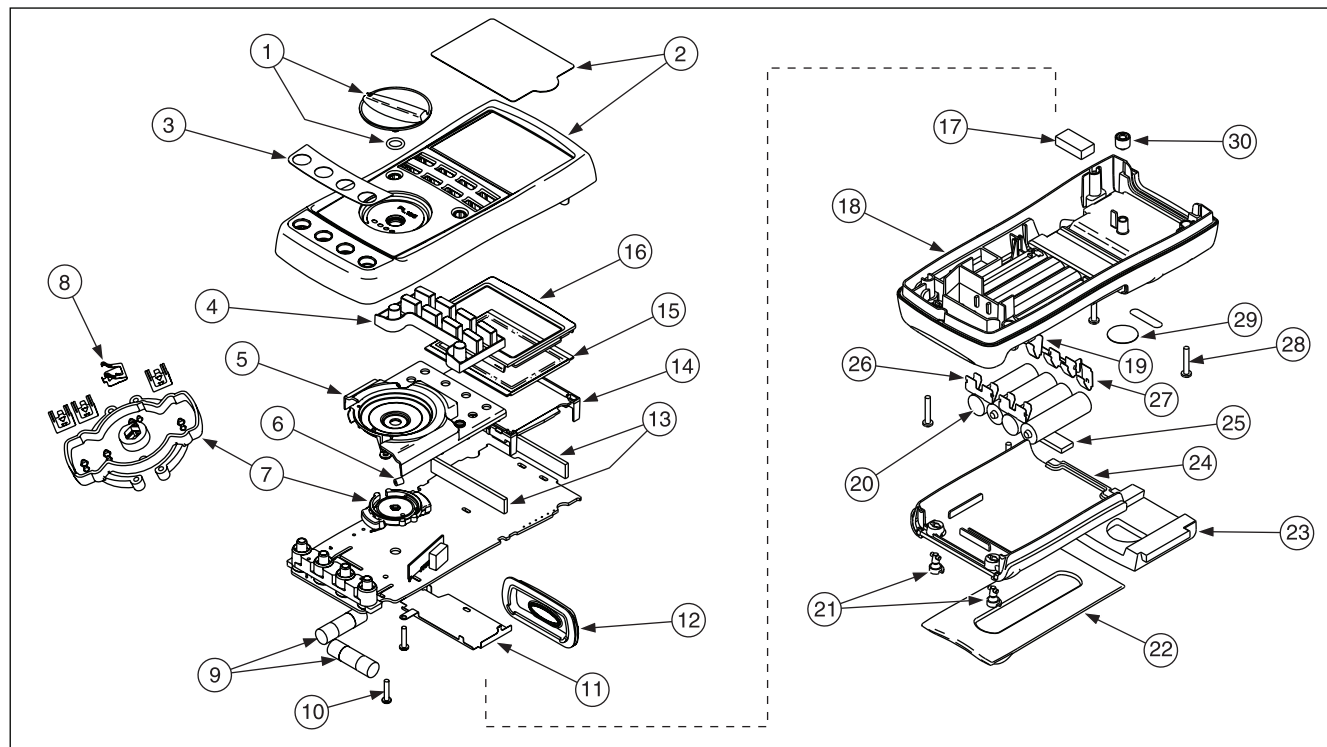
图 12.更换零件
