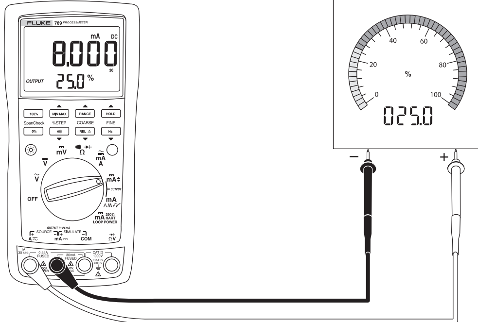
图 7.源电流
