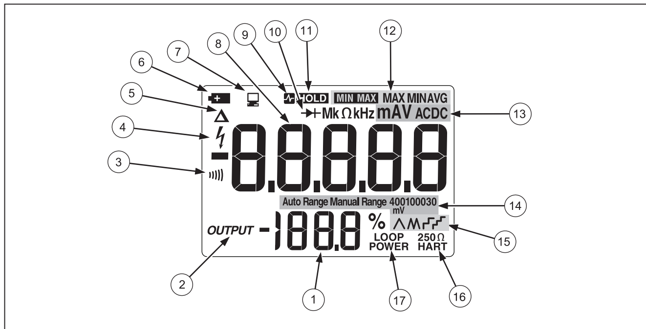
图 6.显示单元
