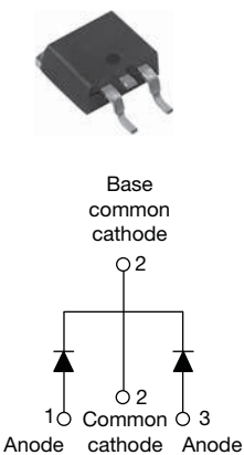
D²PAK
