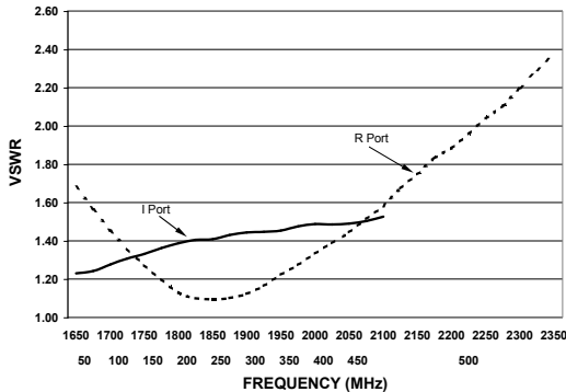
VSWR
