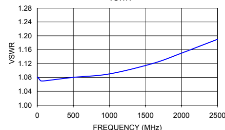
LAT-9+ VSWR
