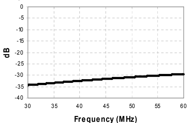
Input Return Loss: Pin6
