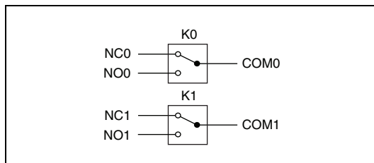
図 3 NI PXI-2599 電源投入時の状態
