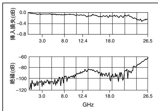
図 1 標準挿入損失および絶縁
