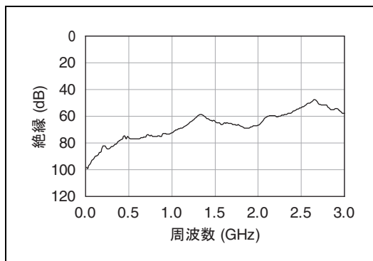
図 4 標準絶縁
