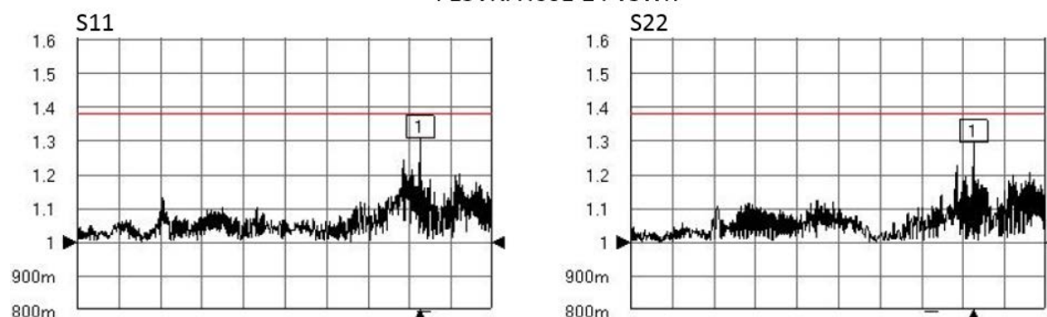
PE3VNA4001-24 VSWR
