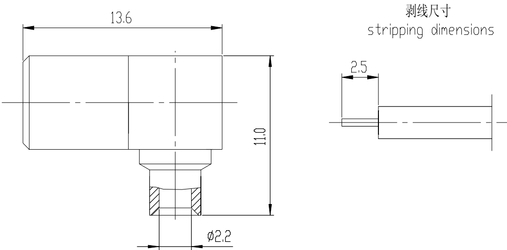
电缆型号:SFT-50-2-1、RG405/U cable type
