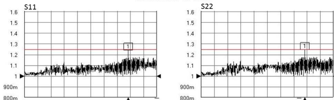
PE3VNA2603-24 VSWR
