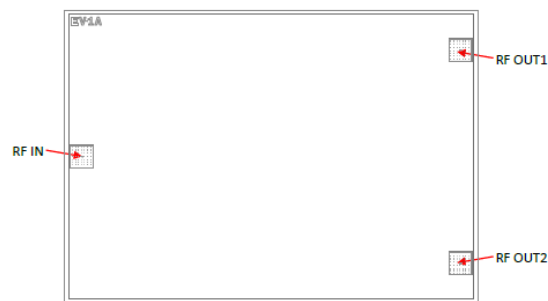
Fig 2. Die Layout
