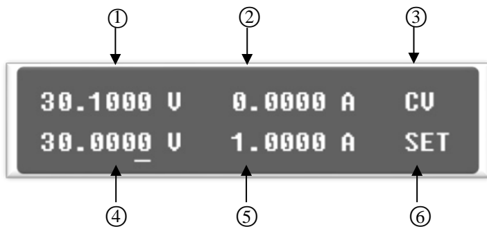
图 5.1-1 VFD 显示屏
