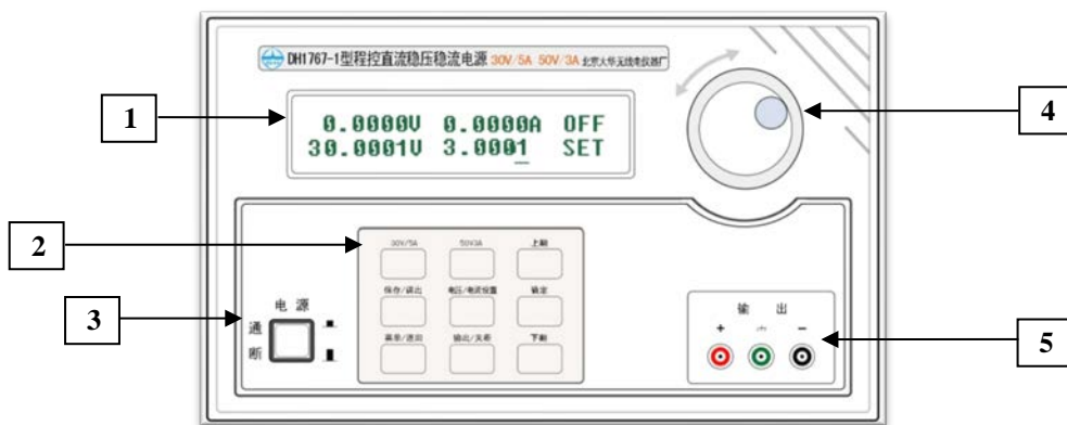
图 5.1 前面板
