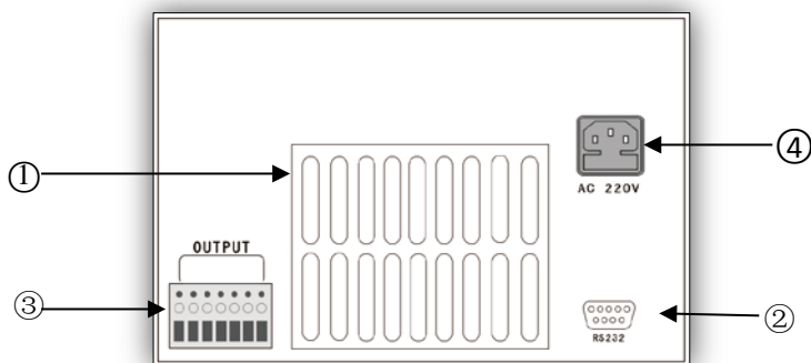
图 5.2-1 后面板
