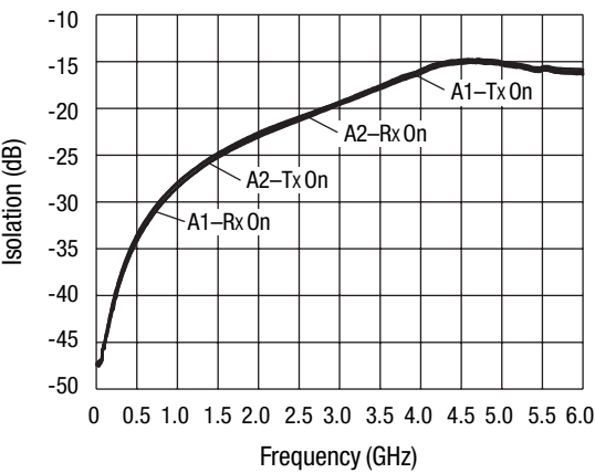
Tx-Rx Isolation
