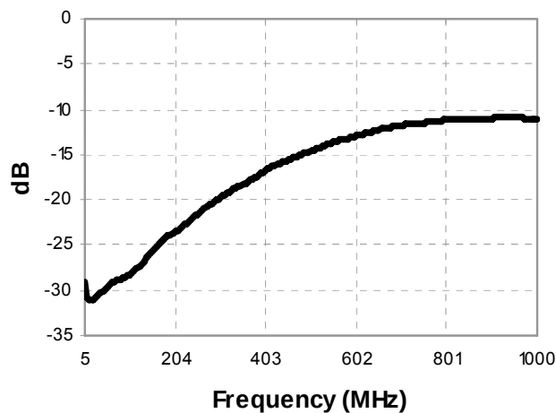
Return Loss: Input (Pin4)
