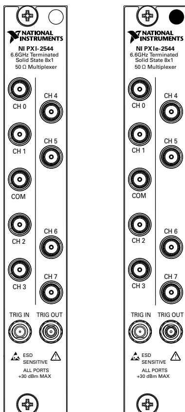
図 5. NI 2544 フロントパネルコネクタ
