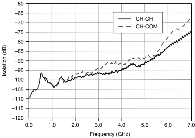
図 3. 標準絶縁
