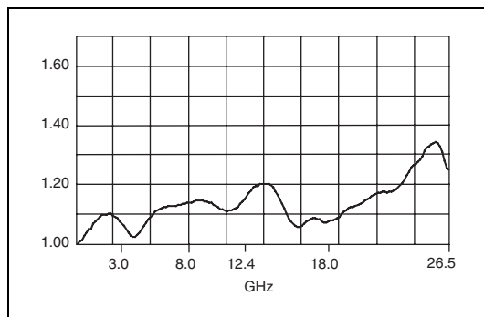
圖 2 標準 VSWR
